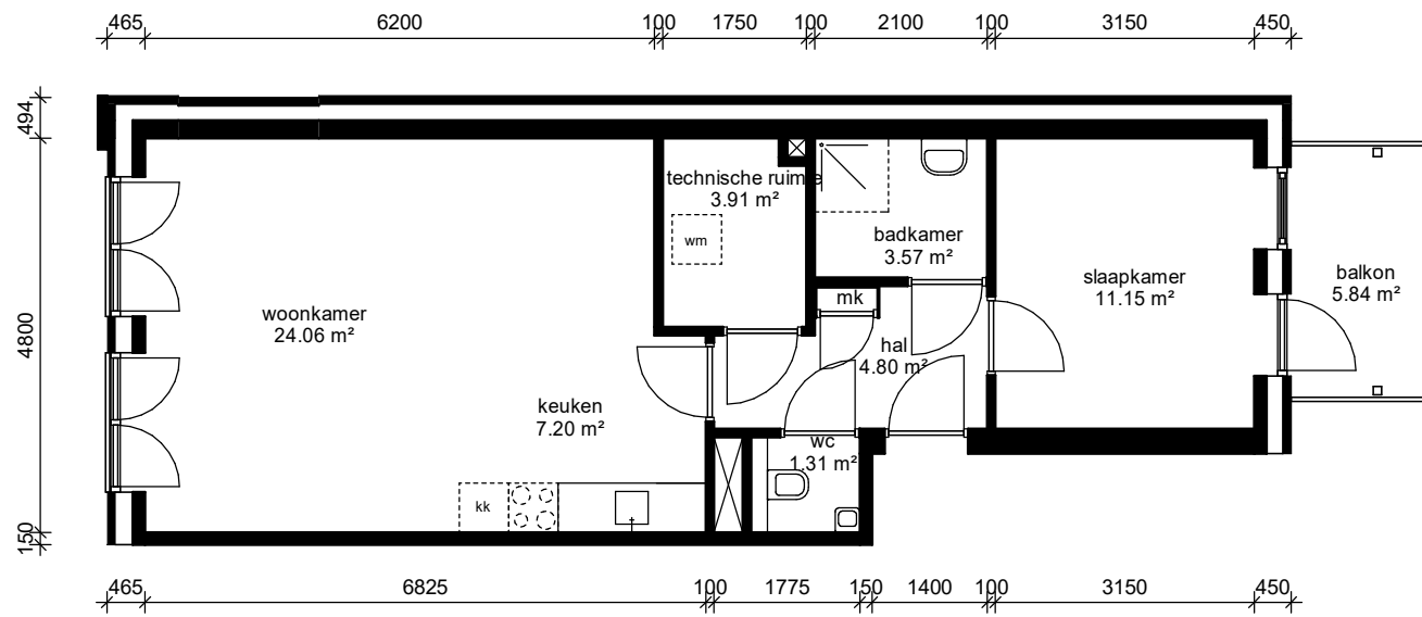
Eerste verdieping
